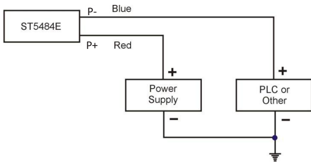
图5: 单个ST5484E地震式变送器的典型安装
