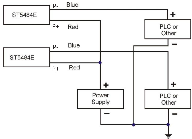
图6: 多个ST5484地震式变送器的典型安装
