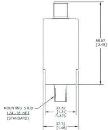
图3: ST5484E-XXX-XX4-XX (MIL-Style 接头) 的外部尺寸。尺寸单位 mm[inches]。0.9 lbs (0.41 kg)
