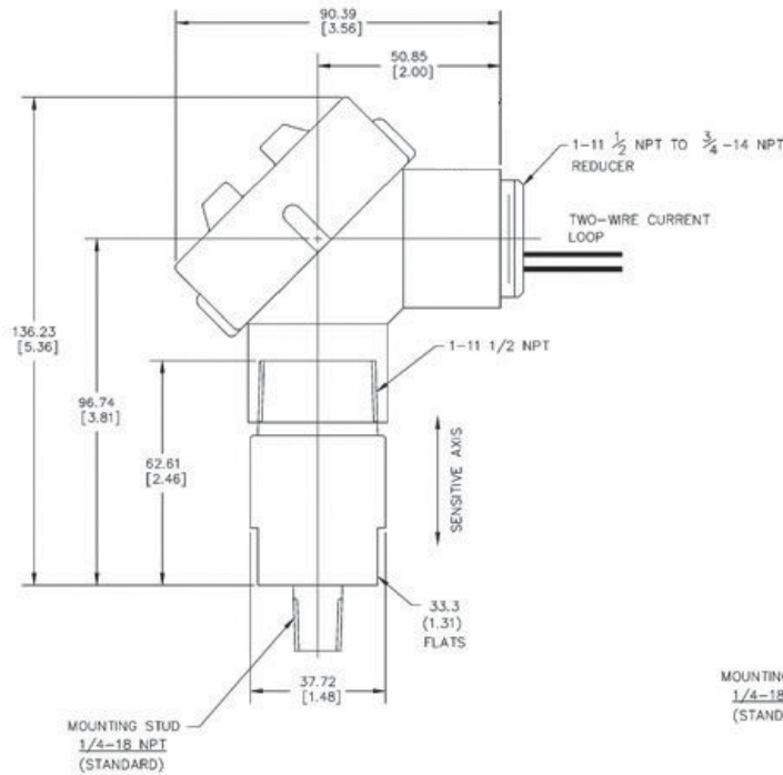
图2: ST5484E的外形尺寸 (所有版本除了MIL-Style 航插接头)。尺寸单位 mm [inches]。可选的* 8200-001 管肘显示已安装。1.55 lbs (0.70 kg)
