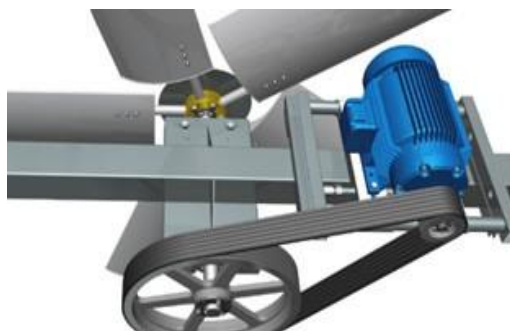
皮带驱动风扇
