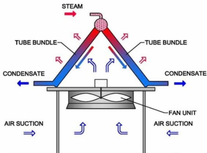
干式冷却塔
