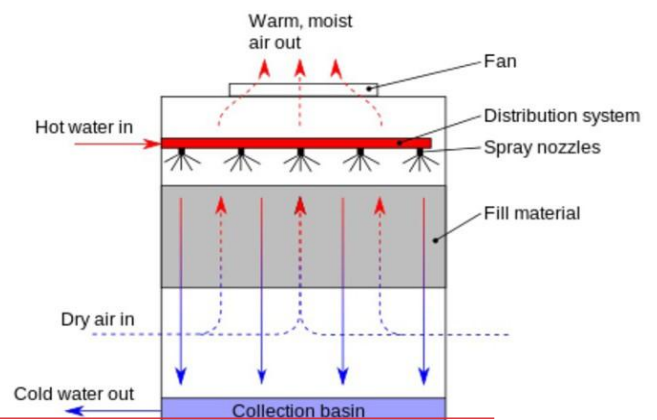
逆流式冷却塔
