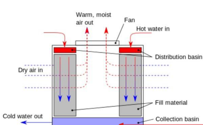
横流（直交流）式冷却塔
