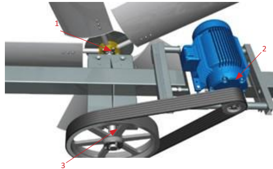
皮带驱动风扇
